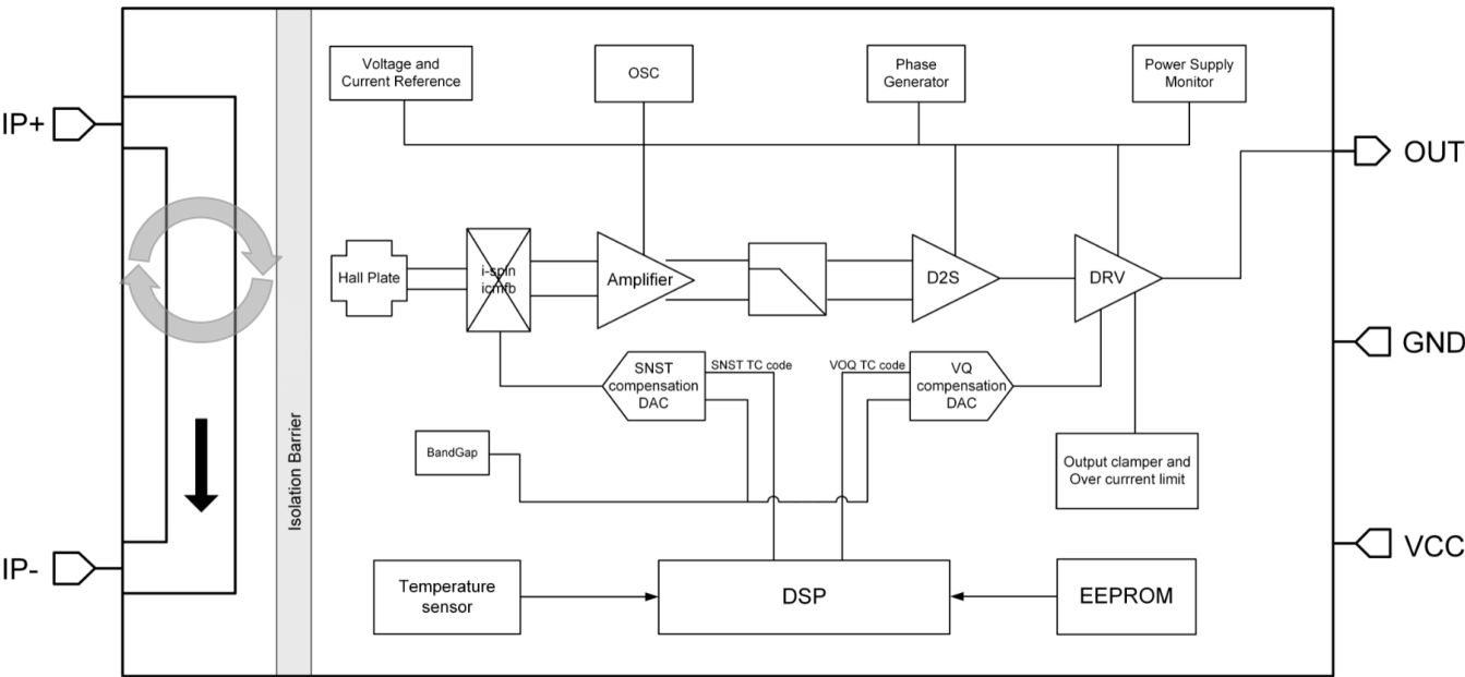
图.1 功能框图
