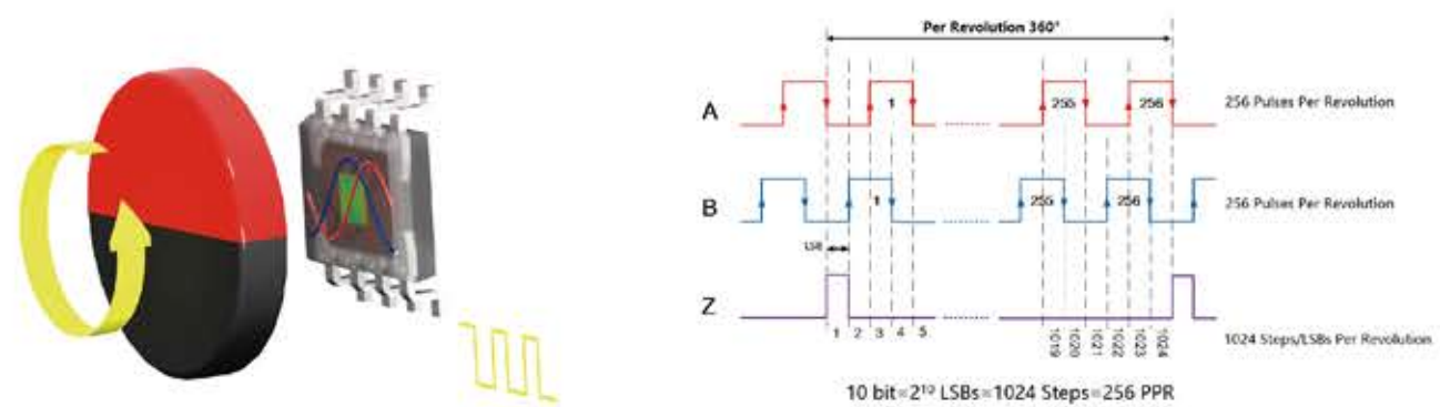
原理图
