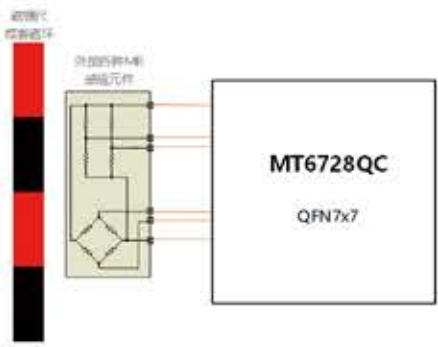
原理图
