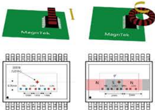
原理图
