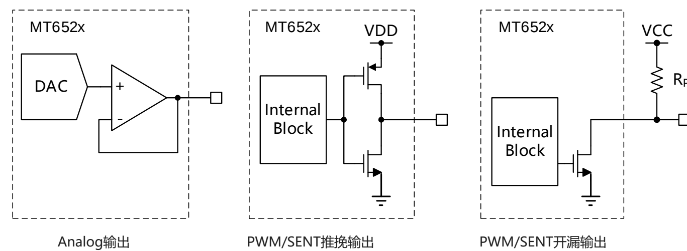
图-6. 模拟输出, PWM/SENT输出的类型
