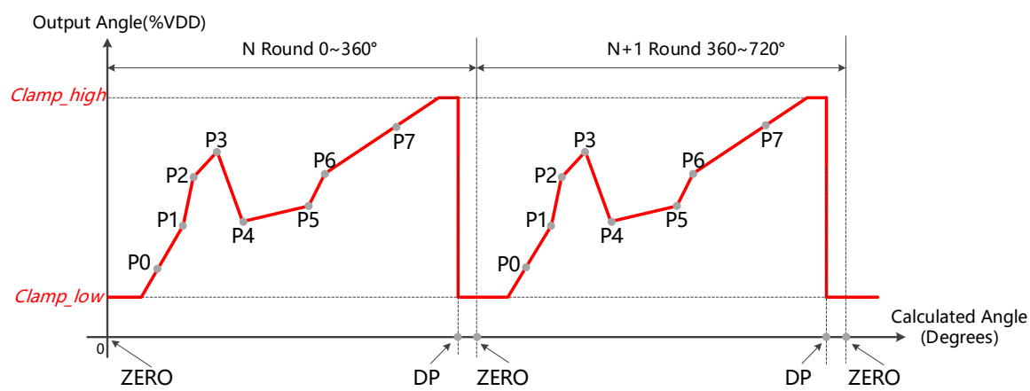
图-23: 输出传递函数（模拟输出、PWM输出、SENT输出）
