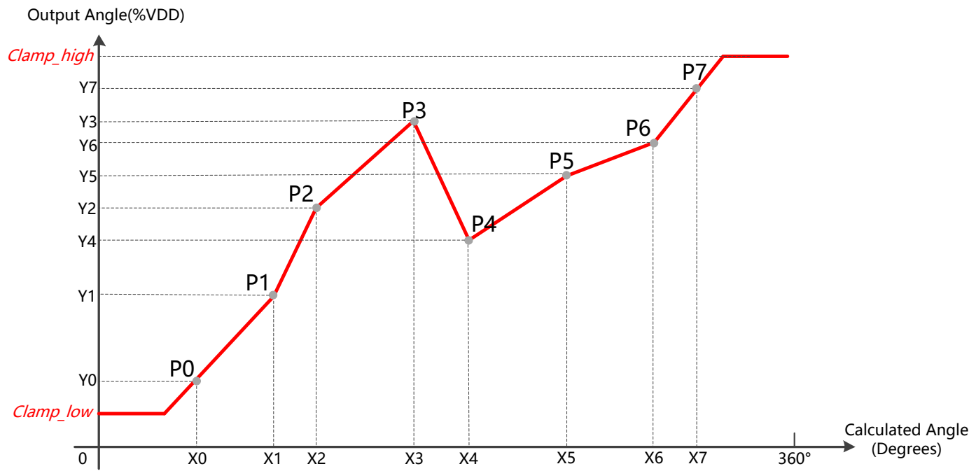
图-25: 输出曲线8点编程（模拟输出、PWM输出、SENT输出）
