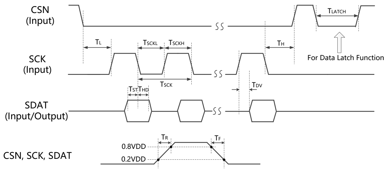
图-11 3线SPI时序图
