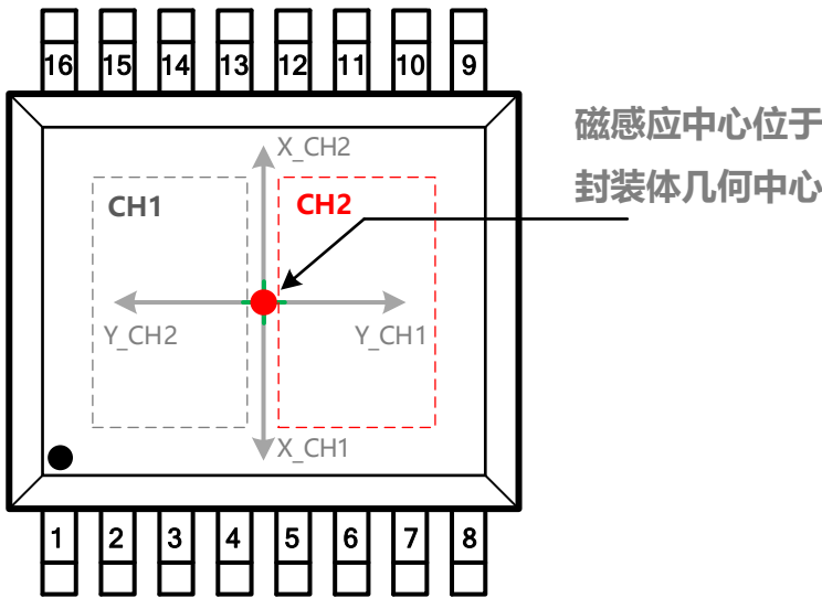
图-2: TSSOP-16 封装 (CH1、CH2为双路芯片每一路的编号)
