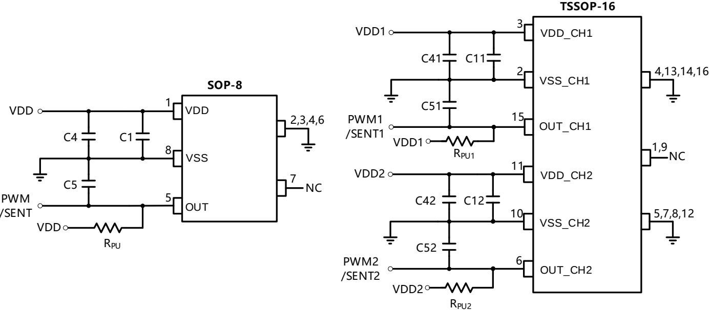
图-30: PWM、SENT开漏输出模式参考电路
