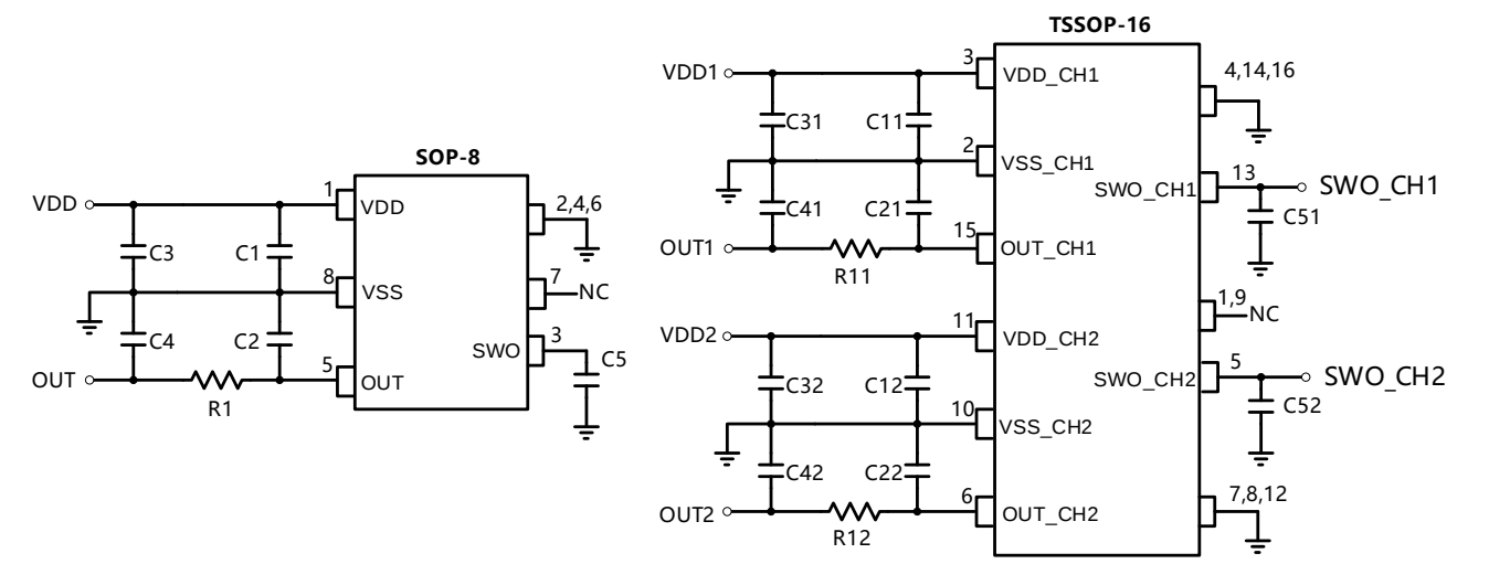
图-28: 模拟输出+开关量输出参考电路
