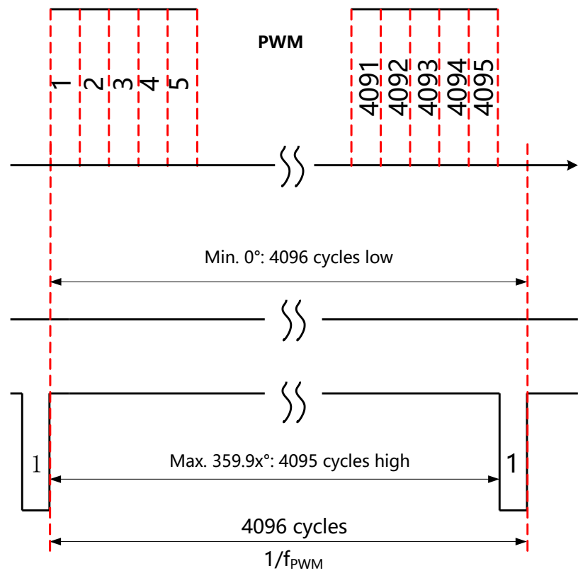
图-9: PWM输出
