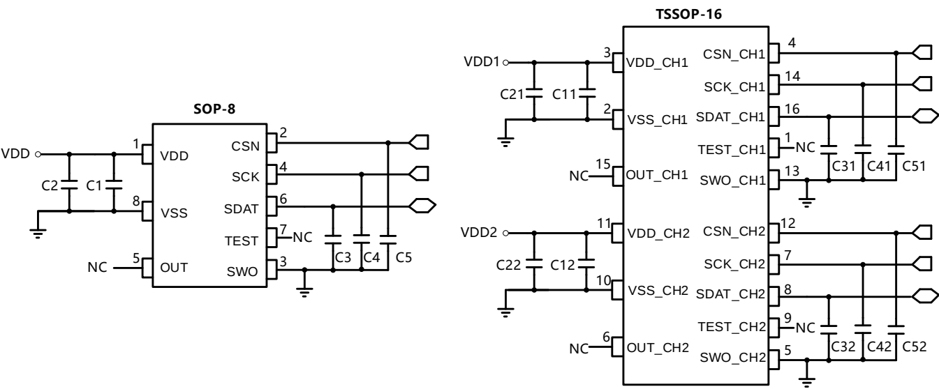
图-31: 3线SPI接口输出参考电路
