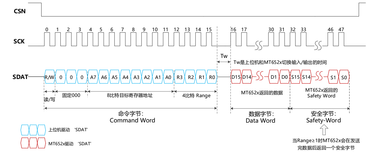
图-12: 3线SPI读操作
