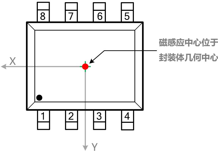
图-1: SOP-8封装
