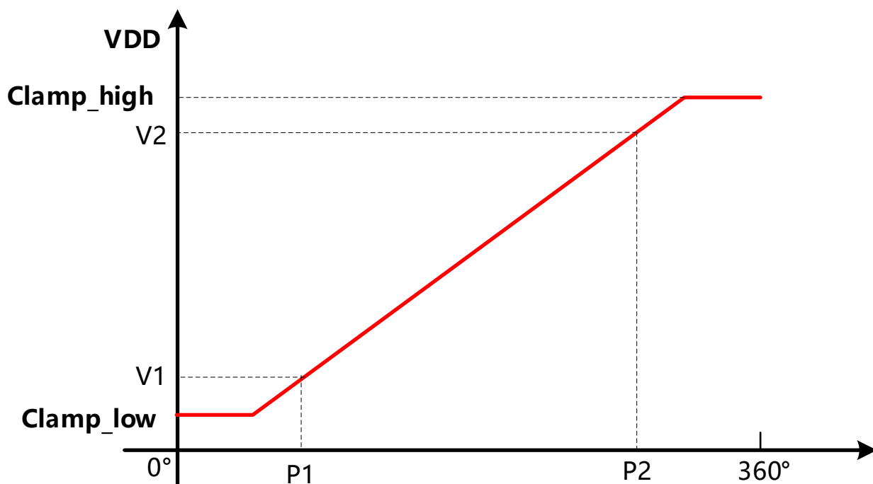
图-7: 模拟输出
