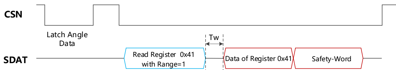
图-17: SPI 读锁存角度数据
